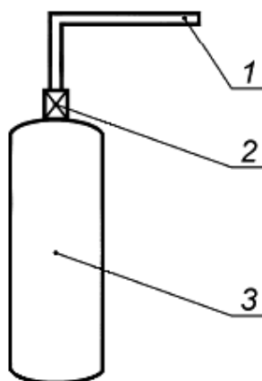
1 - насадок; 2 - ЗПУ; 3 - баллон для хранения компонентов ГПОВ
